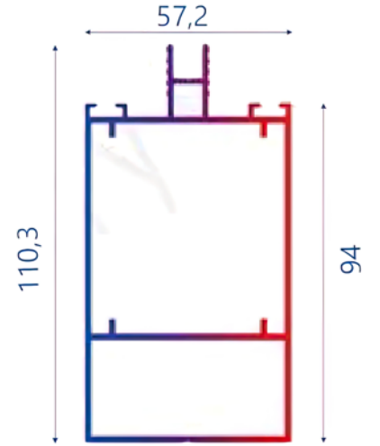
Taşıyıcı Profili 2,079 KG/MT
