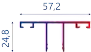
Taşıyıcı Orta Kapak Prf. 0,528 KG/MT
