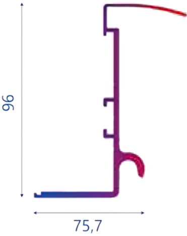
Açı Ayar Profili 1,471 KG/MT
