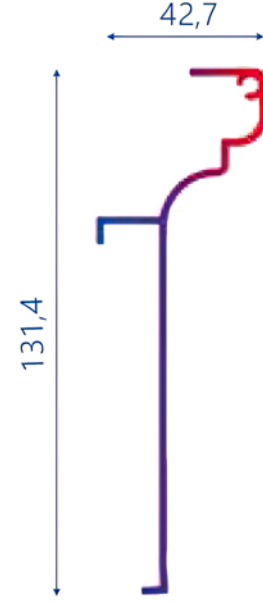
Dekorlu Dere Kapağı 1,057 KG/MT
