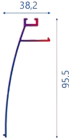
Açı Ayar Kapak Profili 0,595 KG/MT
