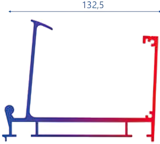
Dere Profi 3,844 KG/MT
